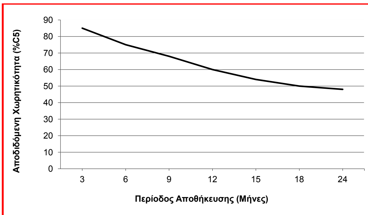
ΔΙΑΓΡΑΜΜΑ II ΑΥΤΟΕΚΦΟΡΤΙΣΗ ΣΕ ΑΠΟΘΗΚΕΥΣΗ ΣΤΟΥΣ 20° C
