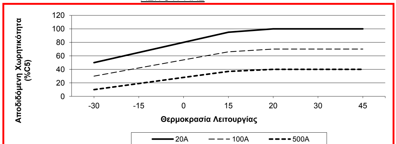
ΔΙΑΓΡΑΜΜΑ I ΑΠΟΔΙΔΟΜΕΝΗ ΧΩΡΗΤΙΚΟΤΗΤΑ ΣΕ ΣΥΝΑΡΤΗΣΗ ΜΕ ΤΗ ΘΕΡΜΟΚΡΑΣΙΑ ΛΕΙΤΟΥΡΓΙΑΣ
